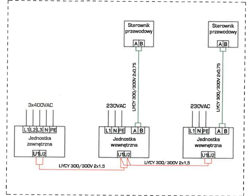
Klimatyzacja - Sala treningowa nr 1/10
