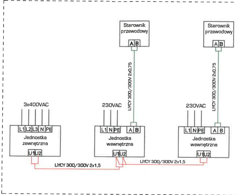
Klimatyzacja - Sala treningowa nr 1/3
