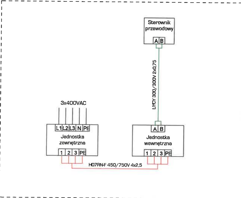
Klimatyzacja - Recepcja
