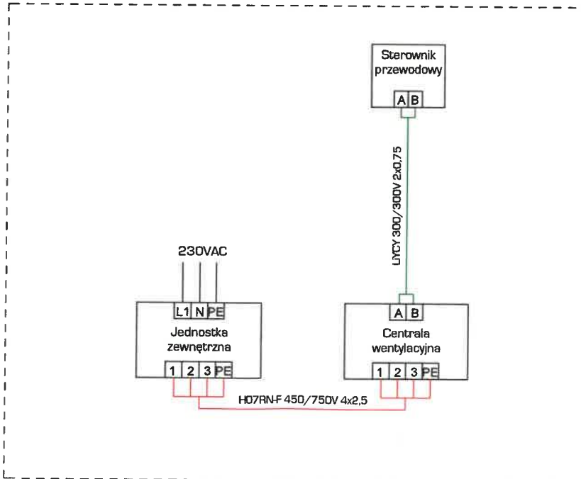
Wentylacja - I system
