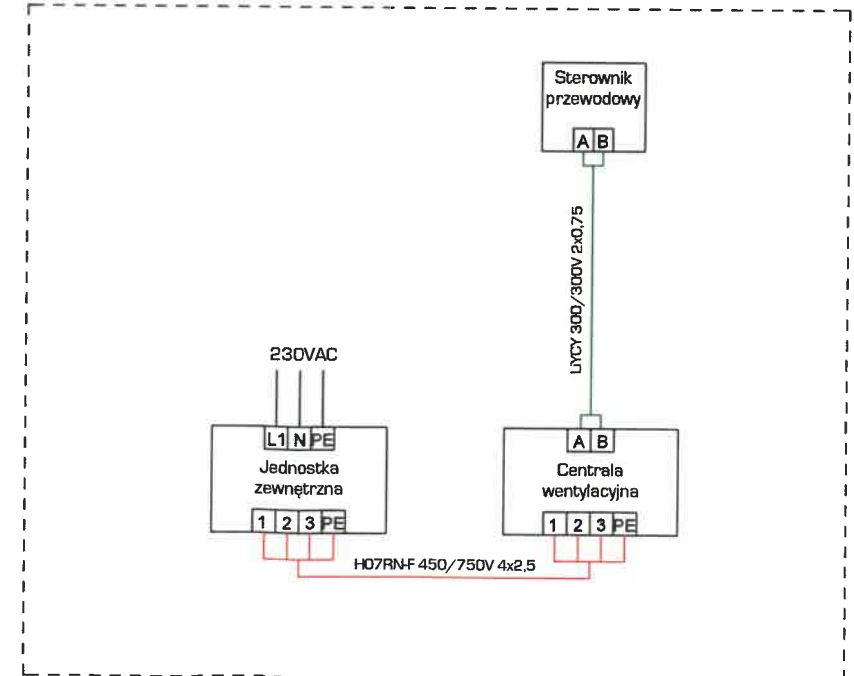
Wentylacja - II system
