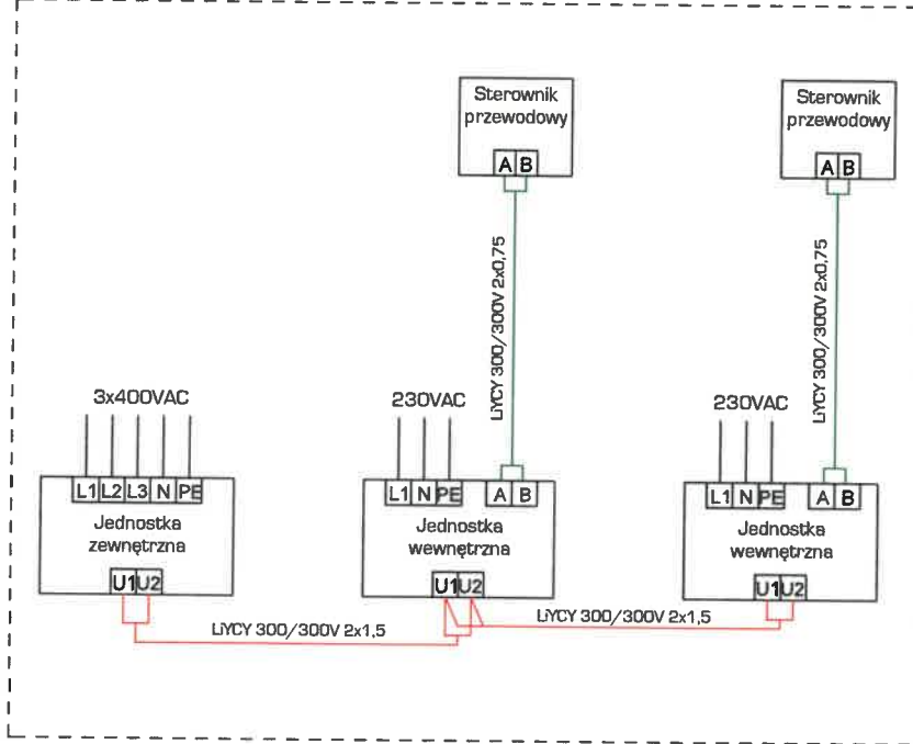
Klimatyzacja - Sala treningowa nr 1/2
